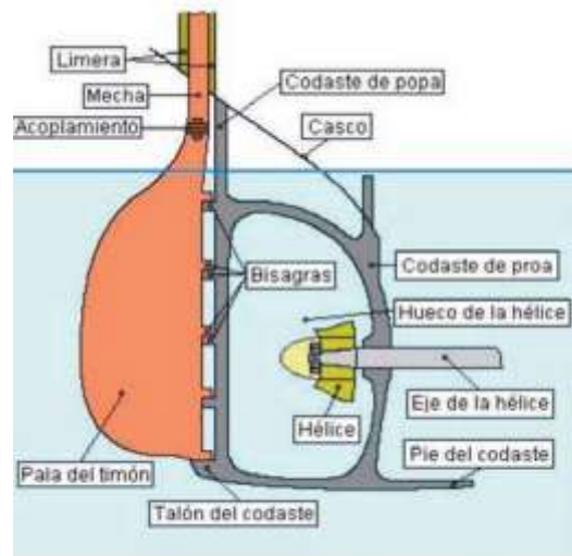
Esquema de un timón actual en una nave a motor.
